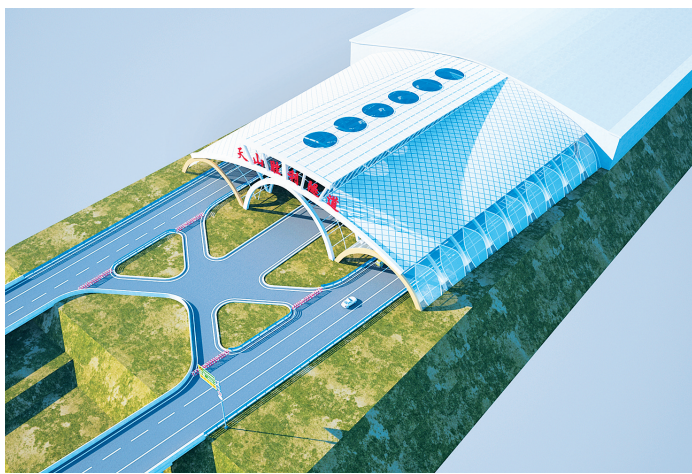
天山胜利隧道钢结构遮光棚效果图。图由乌尉高速6标提供
